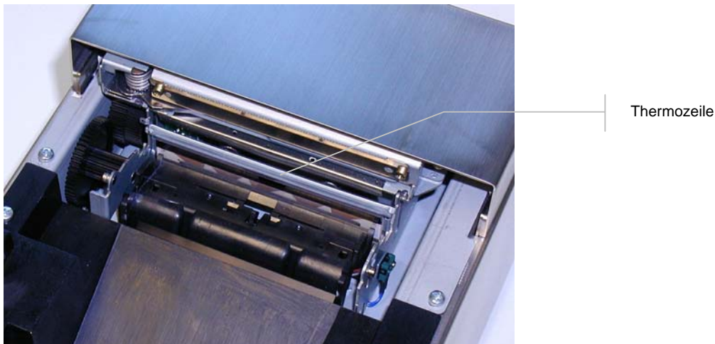
Abb. 6 – Druckwerk
